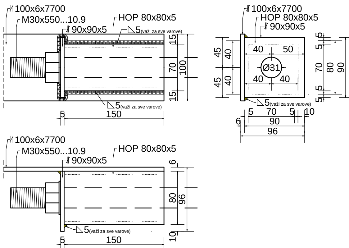
Skica 1. Detalj spoja dve dodatne zatege.
