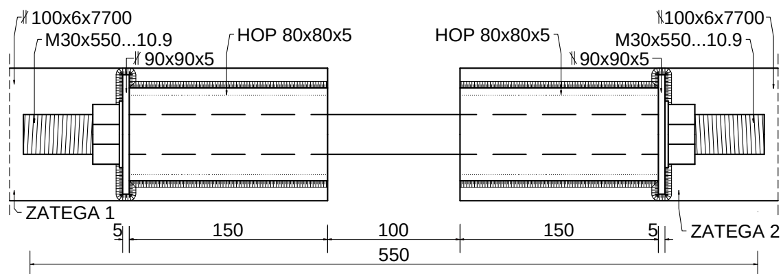
Skica 1. Detalj spoja dve dodatne zatege.
